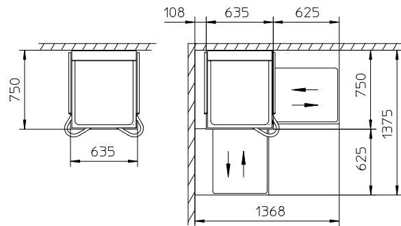
PT-M TwinSet
