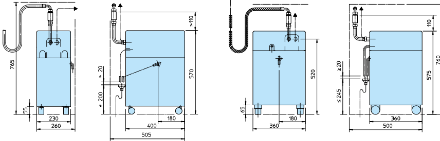
Winterhalter MonoMatik 3
